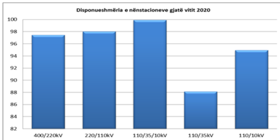
Fig. 3-3. Disponueshmëria e nënstacioneve gjatë vitit 2020
